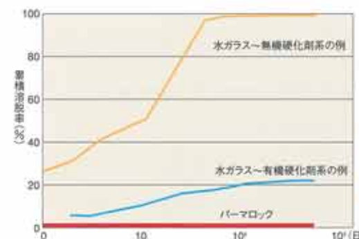
図-6 長期連続透水試験(透水圧49kPa)における各種グラウトのSiO 2 溶脱率 ※49kPa=0.5kgf/cm 2
