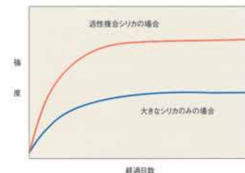
図-7 活性複合シリカ「パーマロック・ASF-Ⅲ」の経時的強度増加の傾向
