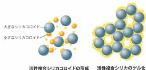
図-3 パーマロック・ASF-Ⅲの反応モデル
